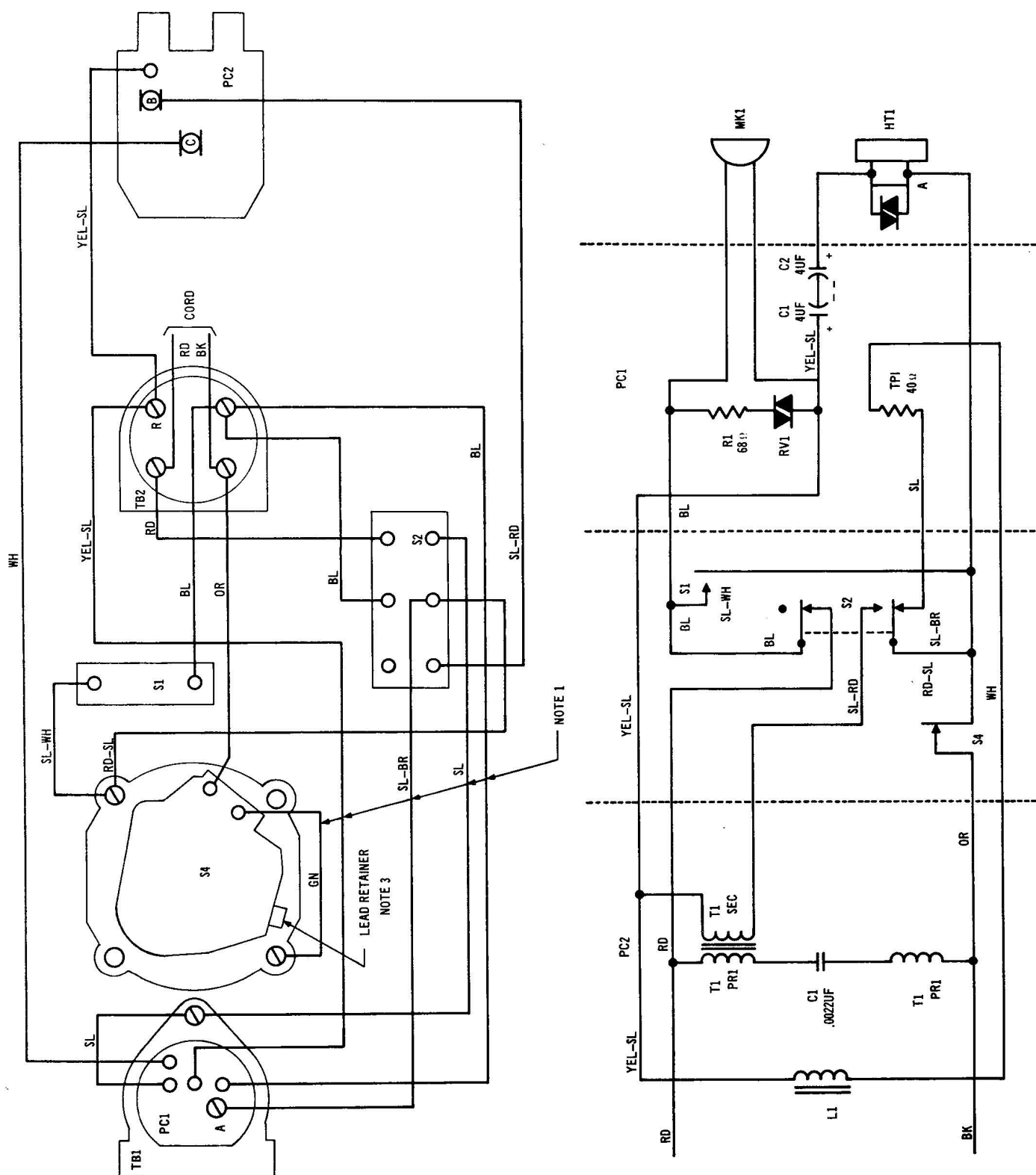
Fig. 4 QSE4B Handset Schematic and Wiring
